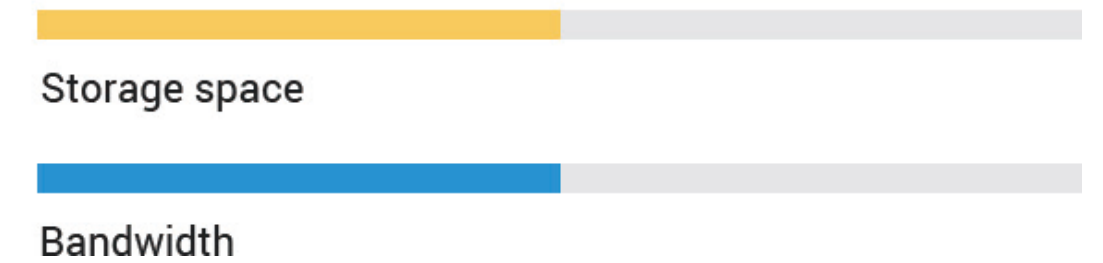
H.265
