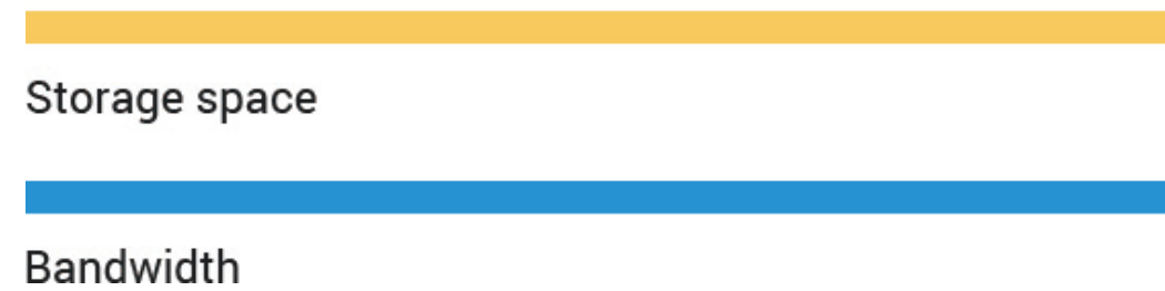
H.264
