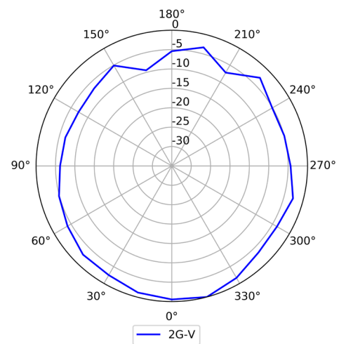
2.4G (Vertical)
