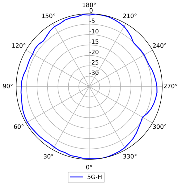
5G (Horizontal)
