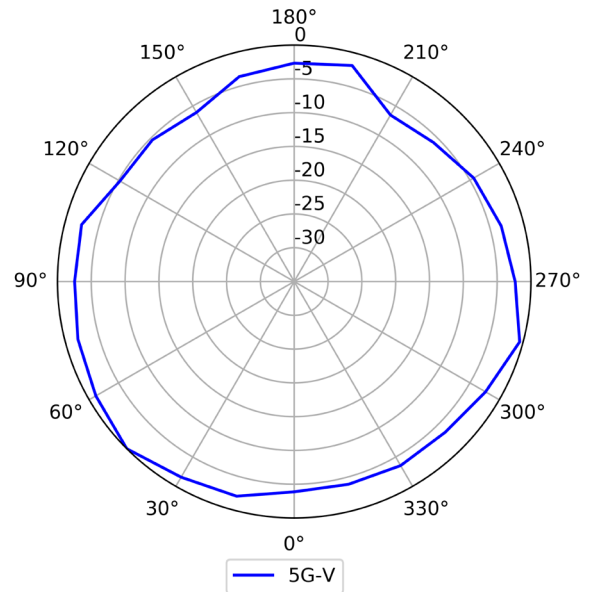
5G (Vertical)
