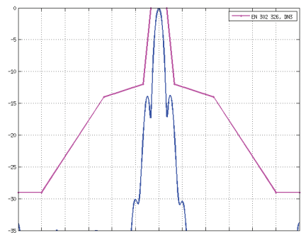
H-Plane Specs
