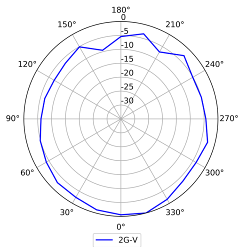
2.4G (Vertical)
