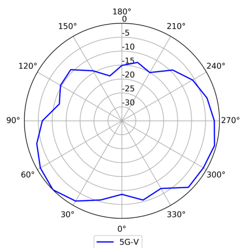
5G (Vertical)
