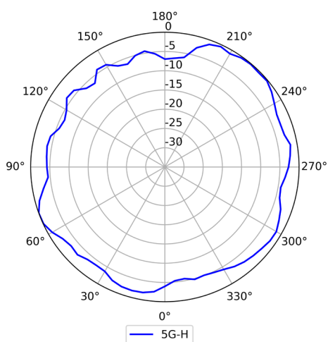
5G (Horizontal)
